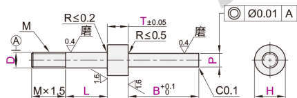
平头型 YHL01/04
