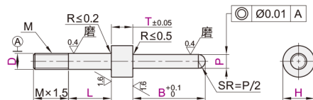
球面型 YHL11/14
