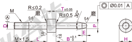
锥角型 YHL31/34
