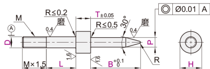
锥头R型 YHL21/24
