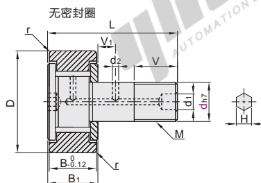
圆柱型 BPF03
