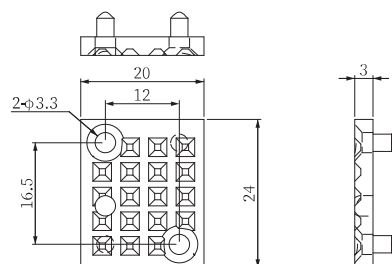
磁性开关 (无触点)
