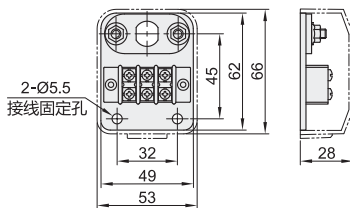
□ 电缆端安装支架(标配件)
