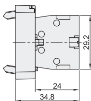
不带灯 ZHC62
