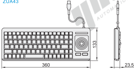
轨迹球 ZUA43
