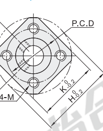
方法兰型 GAF11/12/16
