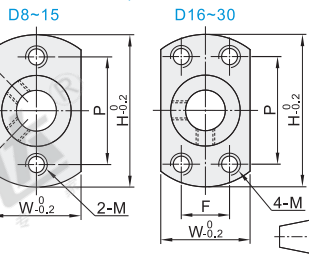
对边法兰型 GAF21/22/26
