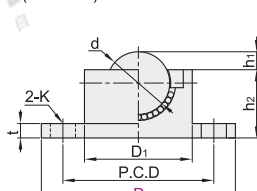
QDA21(SUS304)
