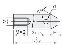
平头锥型 PAJ21/26
