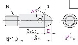
平头锥型 PAJ71/76
