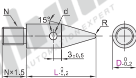
球头锥型 PAJ61/66
