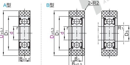
● 圆柱型
