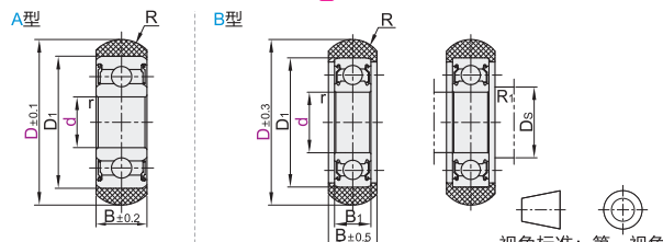
圆弧型
