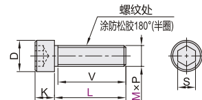
内六角圆柱头螺钉 PACK-TAC16/17/18
