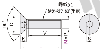
内六角沉头螺钉 PACK-TAU16/17
