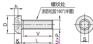
内六角平圆头螺钉 PACK-TAR07/08
