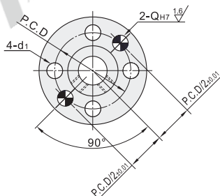
圆法兰型 GAP01/02/06 D12~30
