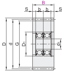
双轴承
