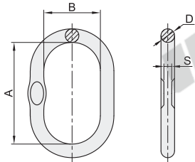
G100锻造强力环 TCE01
