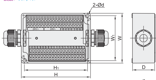
极数: 30P/40P
