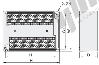
极数: 30P/40P
