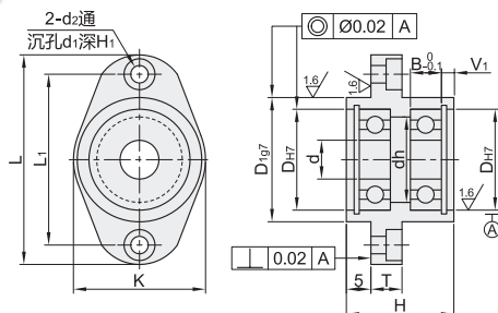
引导型-带挡圈型 E-BFT81/82
