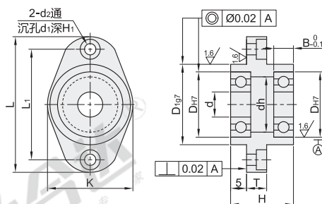
引导型-带挡圈型 E-BFT81/82
