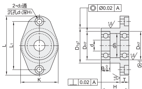
标准型-带挡圈型 E-BFT61/62
