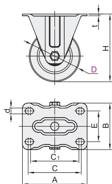
固定型 CFK01
