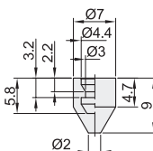
外径D: 7
