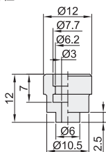
外径D: 12
