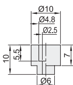
外径D: 10
