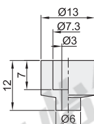
外径D: 13
