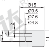
外径D: 15
