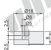
外径D: 18
