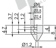
外径D: 6
