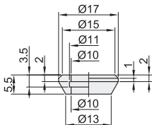
外径D: 17
