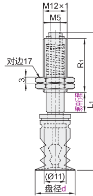
盘径 \varnothing 20
