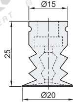
盘径 \varnothing 20
