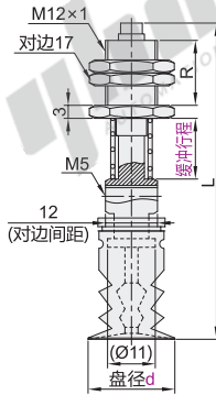
盘径 \varnothing 20
