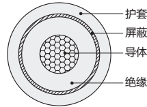
带屏蔽 ZIF37
