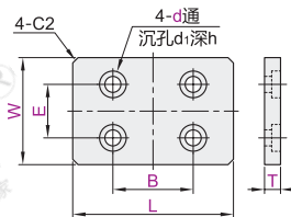
沉孔尺寸表
