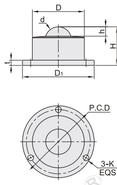
带弹簧向上使用型 QDE34
