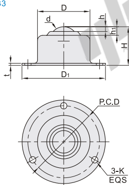
向上使用型 QDE33
