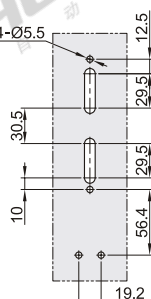
开孔尺寸
