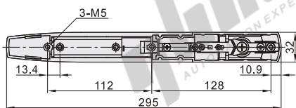
开孔尺寸
