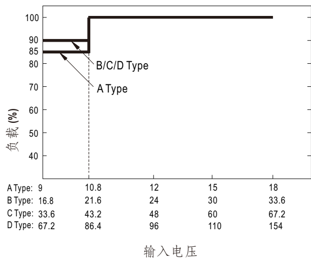
■ 降额VS输入电压曲线
