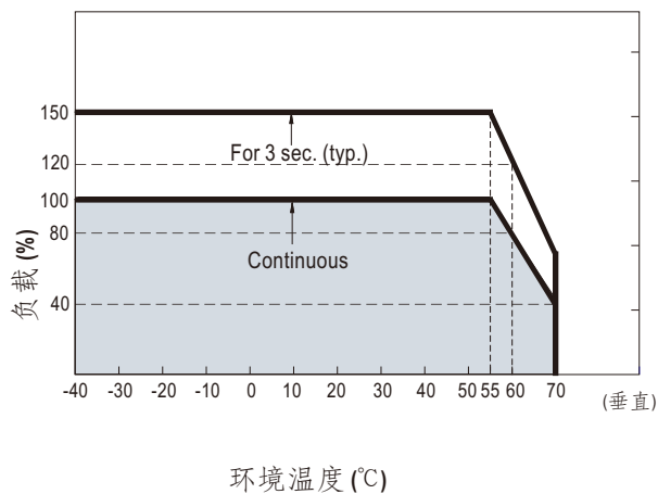
■ 降额曲线
