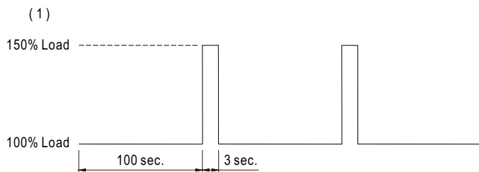
■ 峰值负载曲线
