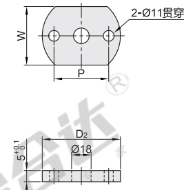
垫片
