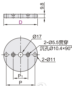
垫片
