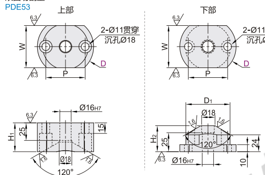
双面切割型
