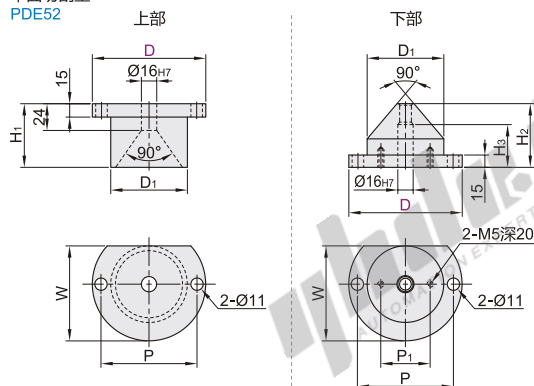
单面切割型
