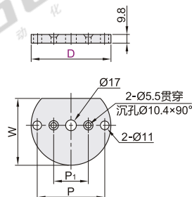
垫片
