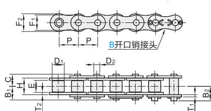
链条 VML01/02/21
