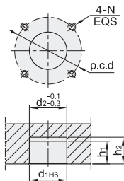
安装孔尺寸
