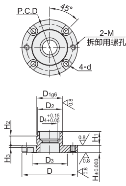
圆柱套 HCD33
