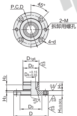
圆锥套 HCD31
