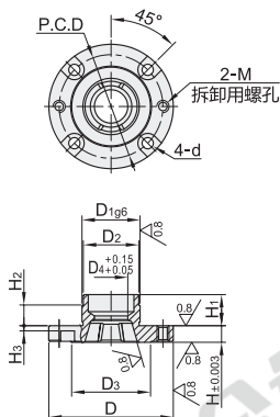
菱形套 HCD32
