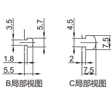
电机安装方式: LD(电机左下折)
