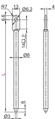
带圆眼连杆 XAV46
