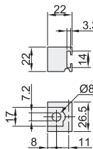
导向件(XAV66-A26.5)
