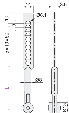
带多孔滚轮连杆 XAV53
