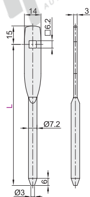
带方眼连杆 XAV47
