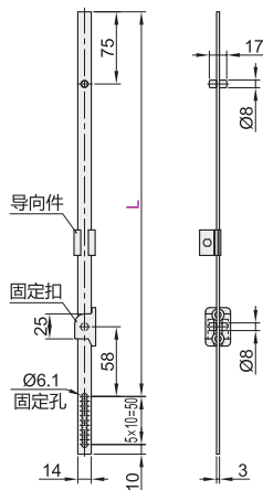
带多孔连杆 XAV54
