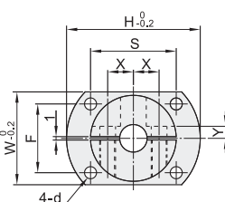
对边法兰型 GAY11/12/16
