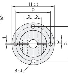
圆法兰型 GAY01/02/06
