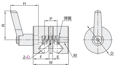
把手型 RDB25/26
