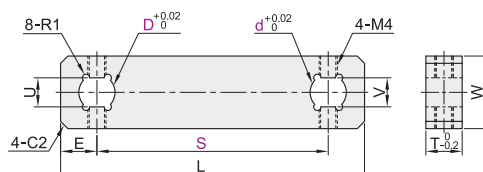
双边止转型 ZFL54/55/56
