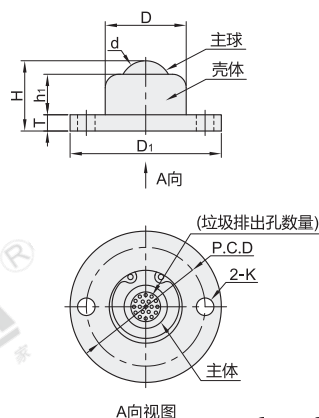
带排出孔型 QFC03
