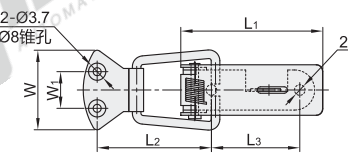
安装孔孔距
