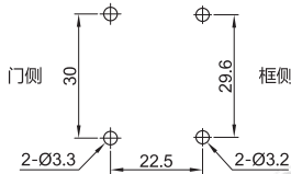
锁闭状态
