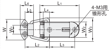
安装孔孔距
