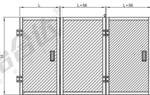
门框开料尺寸
