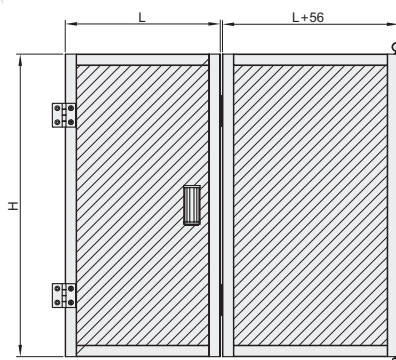
门框开料尺寸
