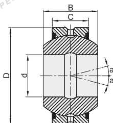
GEG...ES-2RS (两端带密封圈)
