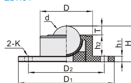
嵌入式 QDH31
