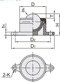
窄耳型 QDH11-25
