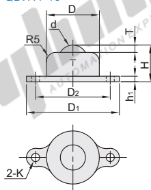
窄耳型 QDH11-16
