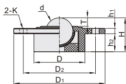
标准型 QDH01
