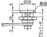
内六角形锁芯 XAS09/10
