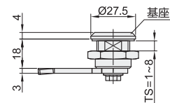
四方形(带槽) 锁芯 XAS08
