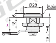
一字形(带防尘)锁芯 XAS70
