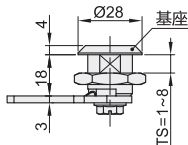
内六角形锁芯 XAS12
