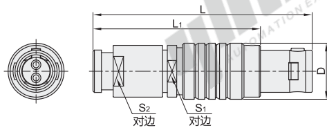
直通型插头 ZIX83
