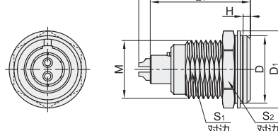
后螺母插座 ZIX84
