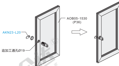
分解图
