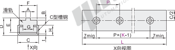
凸型双排 VSW03/04/23/24
