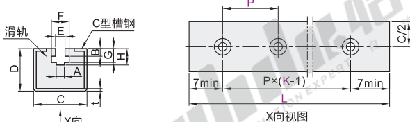
凹型单排 VSW06/07/26/27
