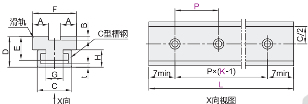
凹型单排 VSW06/07/26/27
