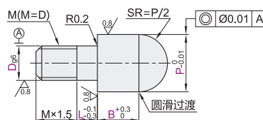
外螺纹型 YFC77/78
