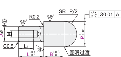
内螺纹型 YFC75/76
