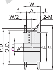
带轮形状 A形
