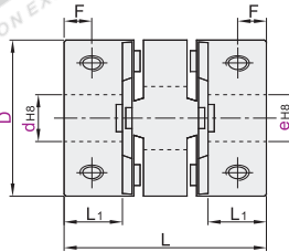
双膜片 DBA13
