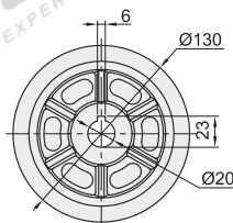
键槽孔型 CNG11
