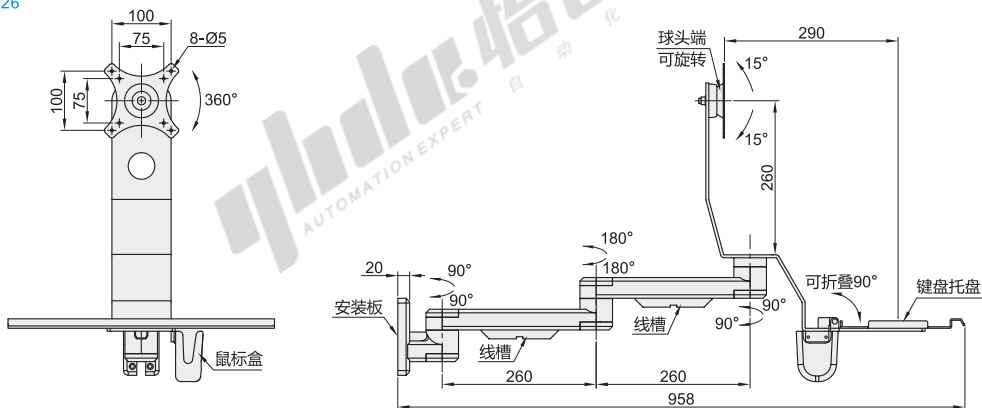
安装板尺寸
