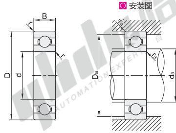
安装图
