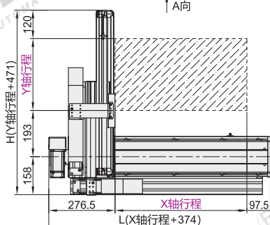
X轴尺寸
