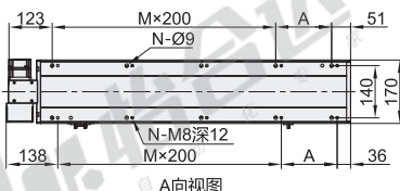
X轴尺寸
