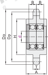
双轴承 VLS12
