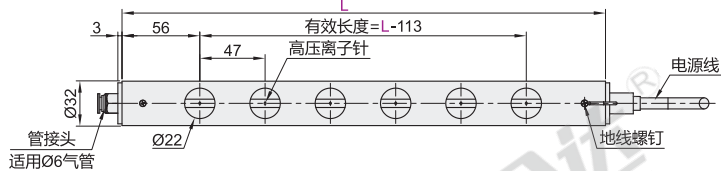
气源型 ZWF16/17
